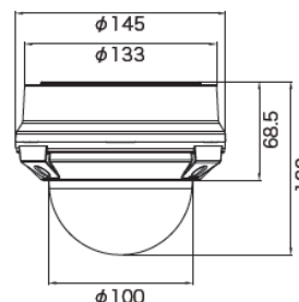
外形図(mm)
