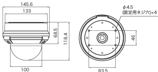
外形図(mm)
