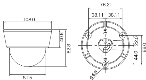
外形図(mm)
